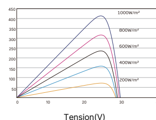
Courbes P-V du Module PV (420W)
