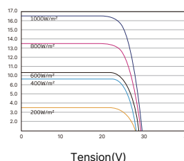
Courbes I-V Du Module PV (420W)
